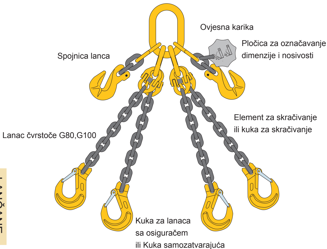
Komponente lančane priveznice - 6;7;8;10;13;16;18;20;22;26mm
